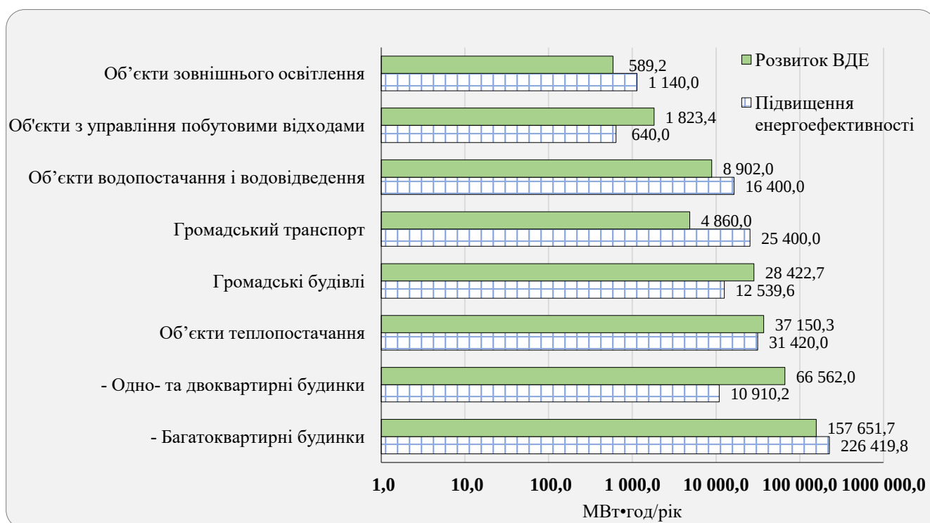
Рис. 6.1 Очікувані результати впровадження заходів МЕП в розрізі секторів (абсолютні значення, логарифмічна шкала)
