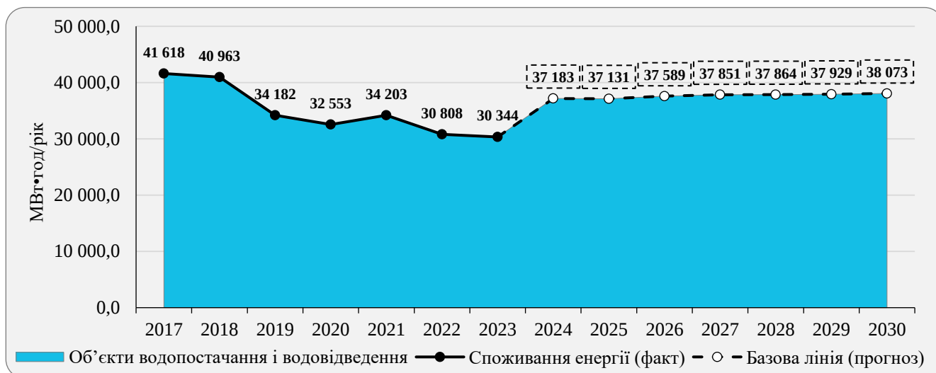
Рис. 3.8 Фактичне та прогнозне споживання енергії об'єктами водопостачання та водовідведення (2017-2030)
